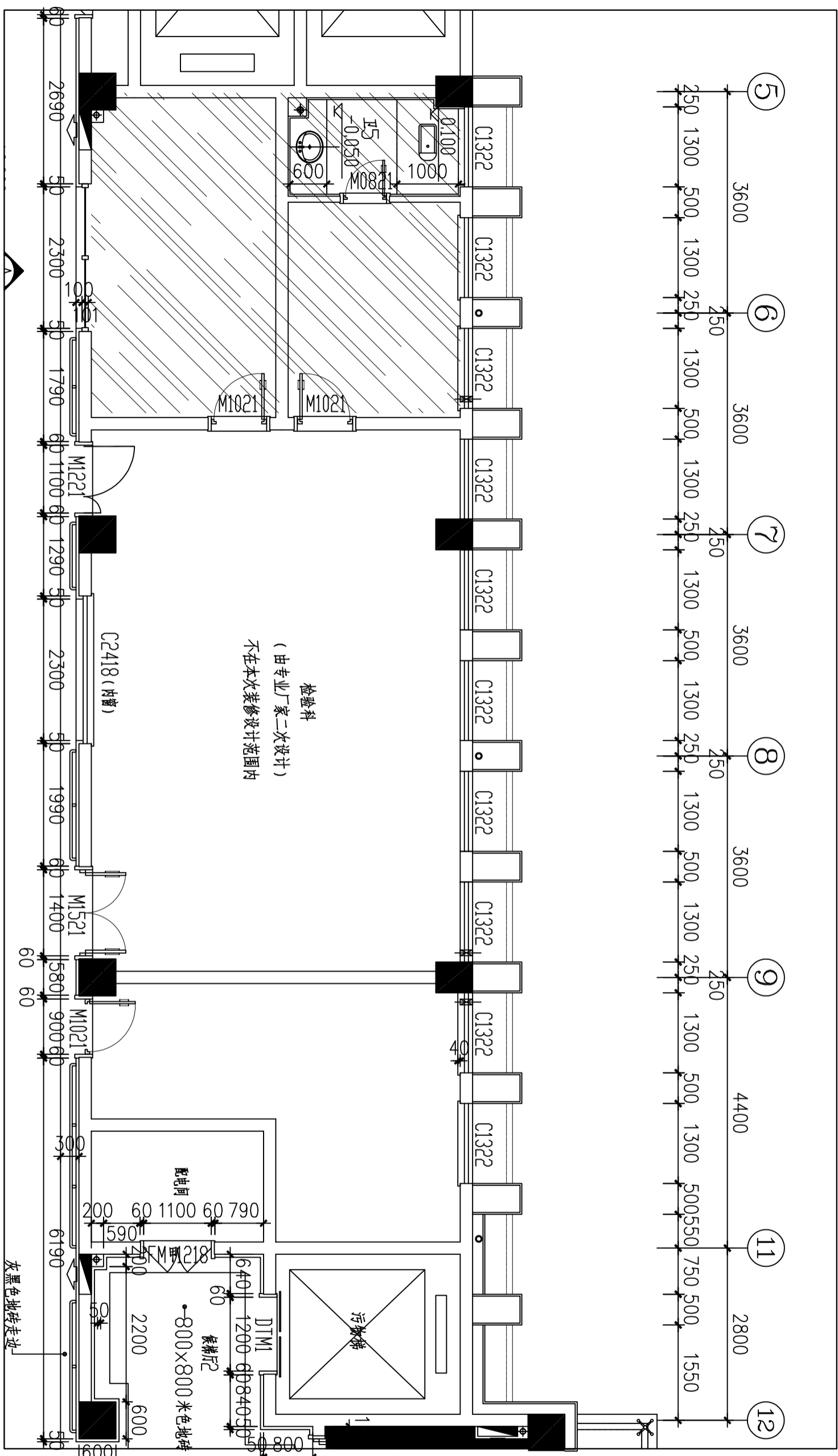
原始结构平面图
